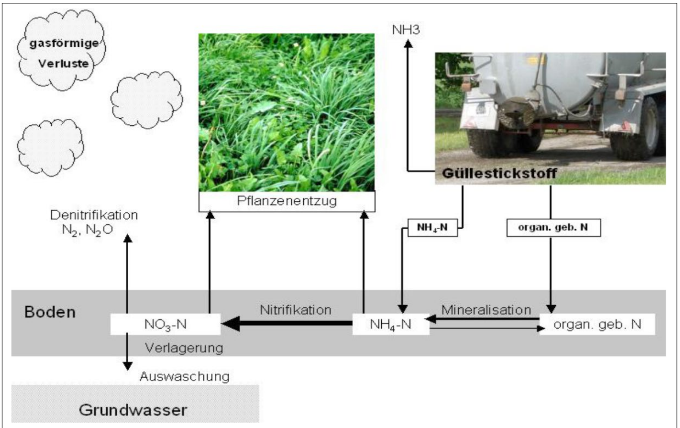
Abb. 1: Stickstoffkreislauf
